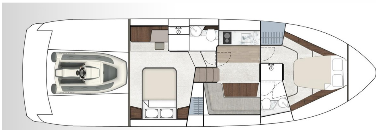
Нижняя палуба, 2 каюты (мастер-каюта на миделе)
