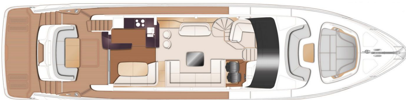
Главная палуба
