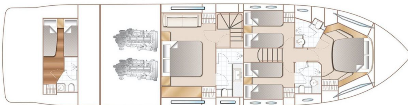
Нижняя палуба
