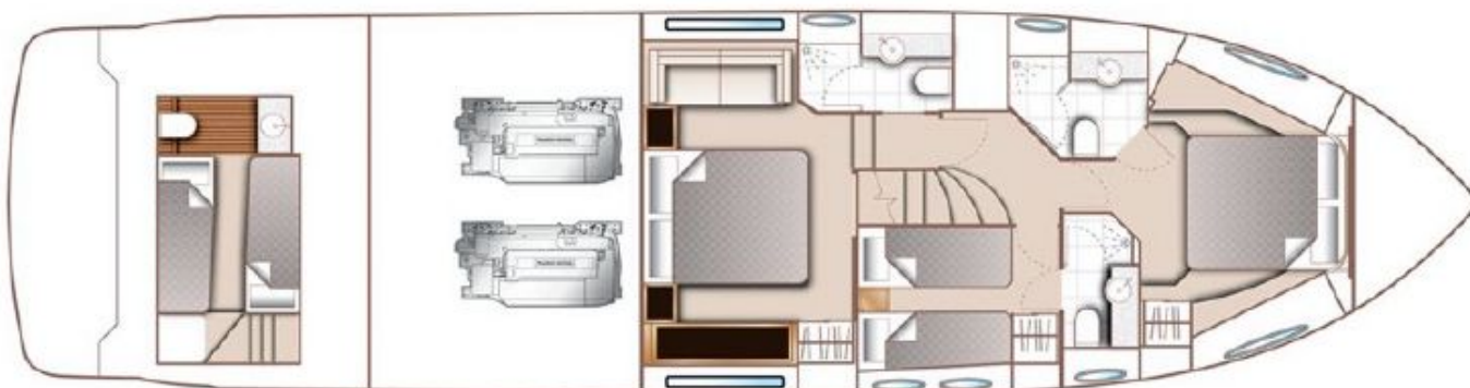
Нижняя палуба
