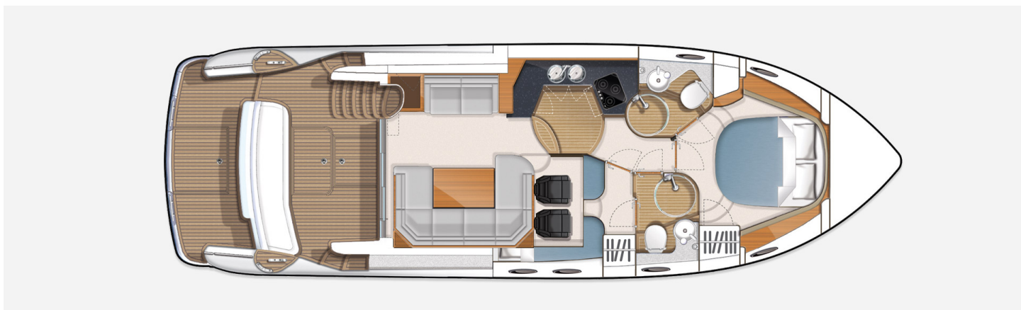
Главная палуба
