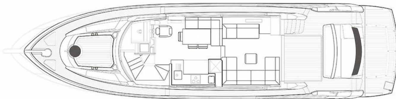
Главная палуба
