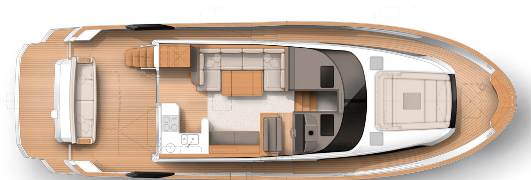
Главная палуба
