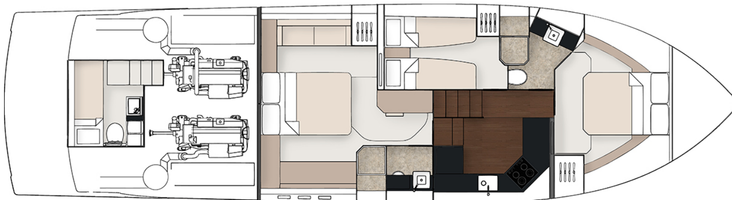
Нижняя палуба, три каюты с камбузом
