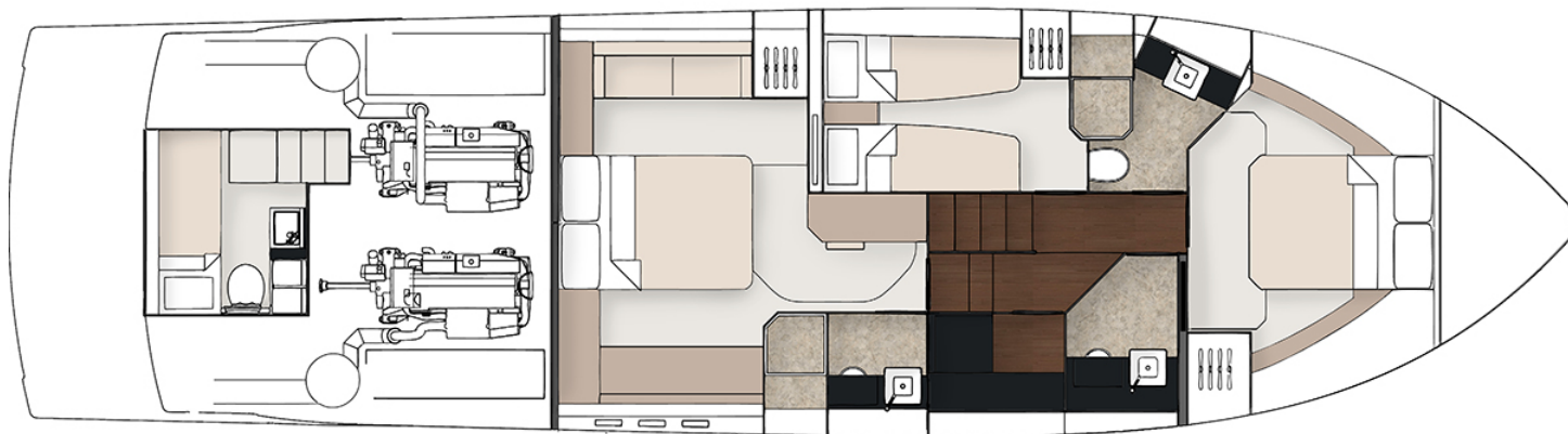
Нижняя палуба, три каюты с дневным санузлом
