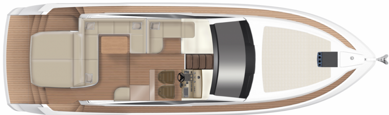
Главная палуба
