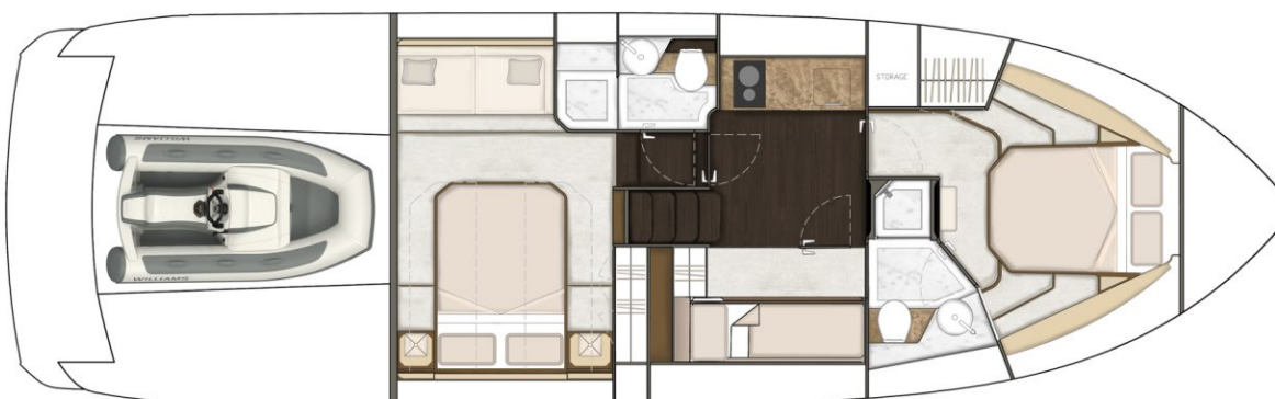
Нижняя палуба, 3 каюты (мастер-каюта на миделе)
