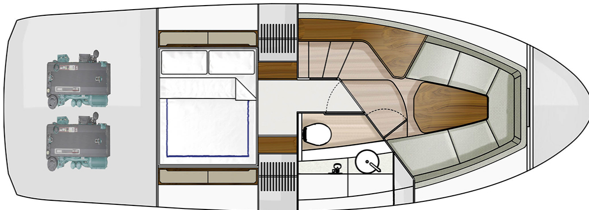
Нижняя палуба
