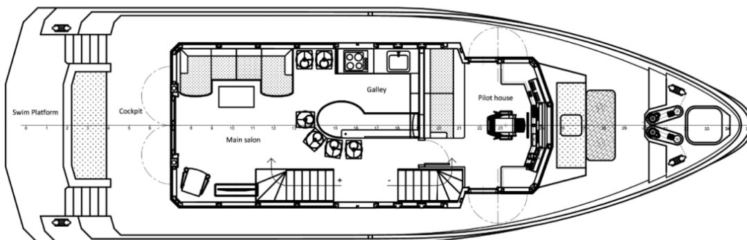
Главная палуба
