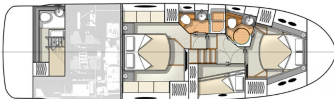
Нижняя палуба
