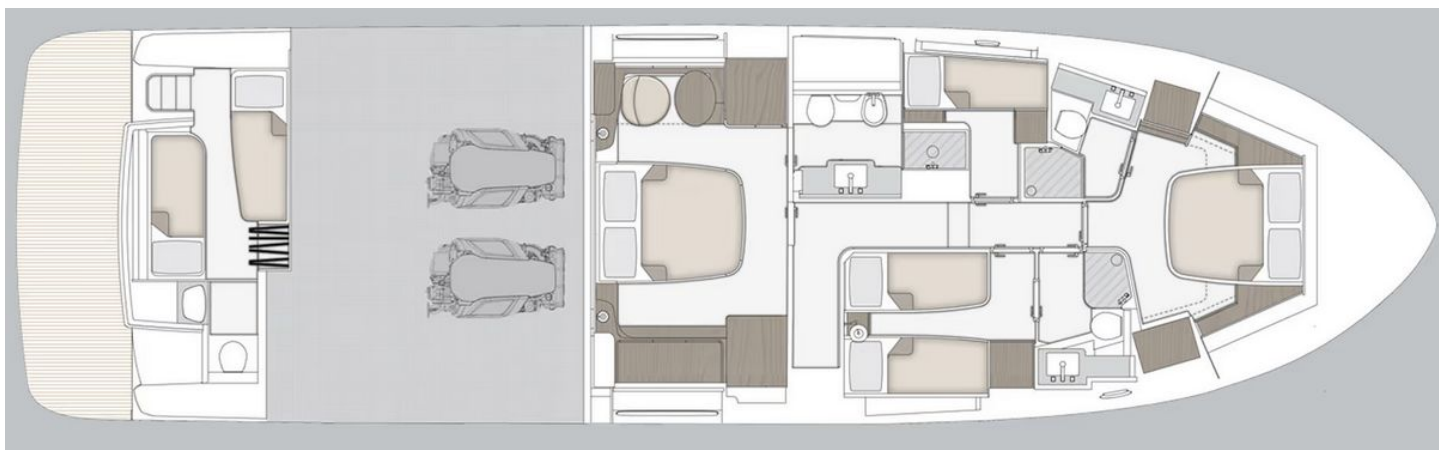
Нижняя палуба
