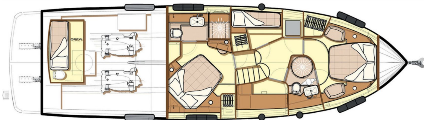
Нижняя палуба
