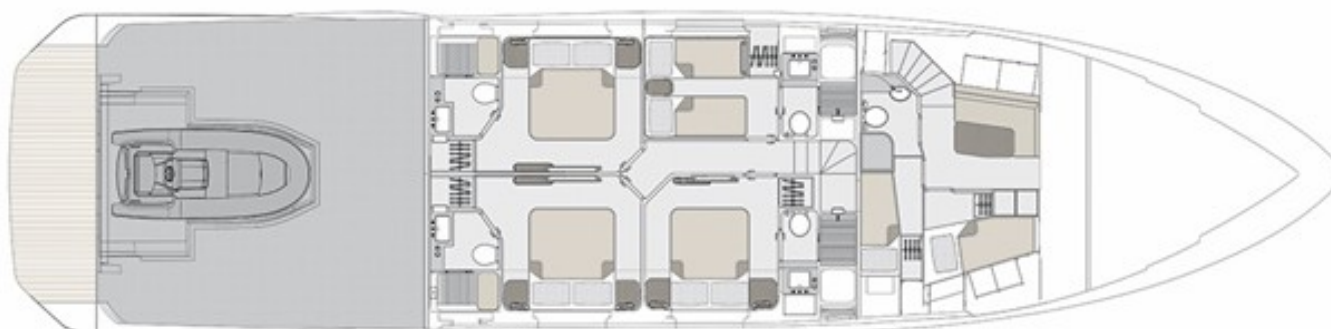
Нижняя палуба
