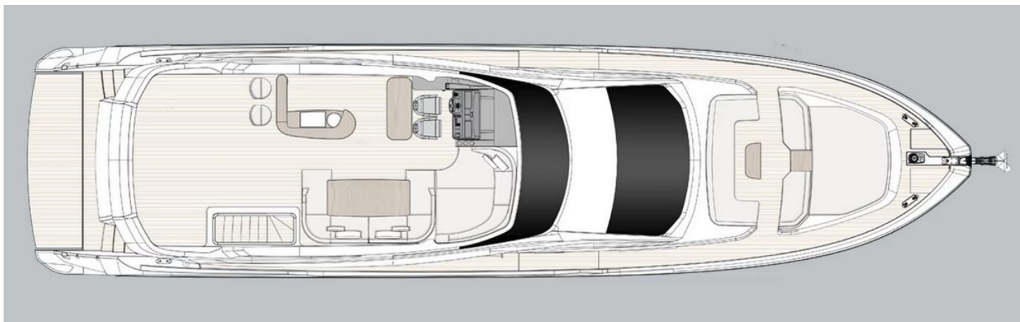
Главная палуба
